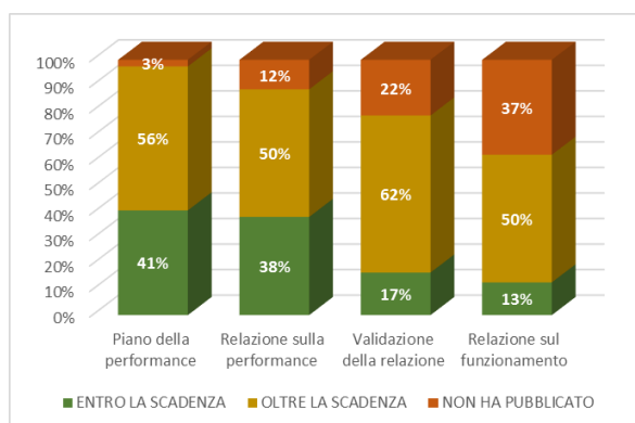
Figura 2 - Pubblicazione documenti
